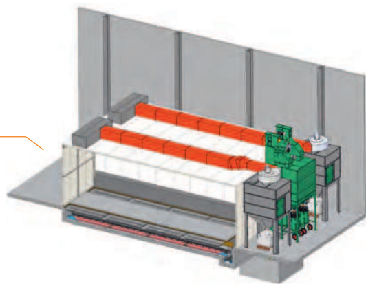
Strahlhalle ausgelegt für zwei verschiedene Strahlmittel mit automatischer Magnetabscheidung und Aufbereitungsanlage
